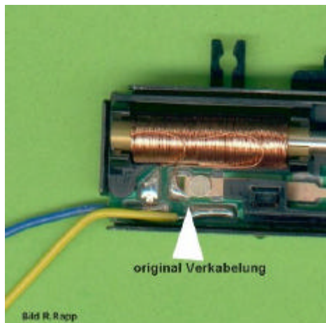
Original Verkabelung
