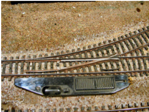
Typ 1 mit Laterne Hohlprofil
