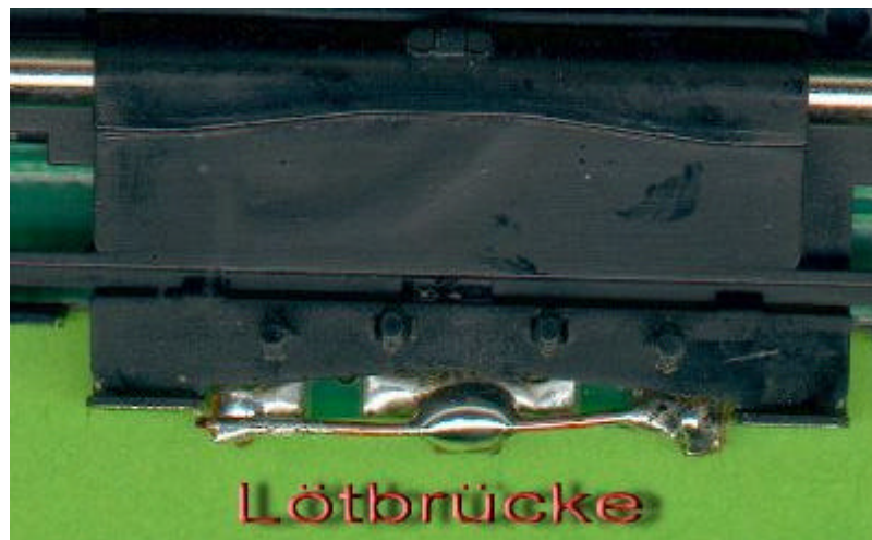
der umgebaut Digitale Weichenantrieb durch eine Lötbrücke
